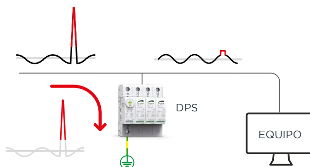
Principio de funcionamiento de un DPS
